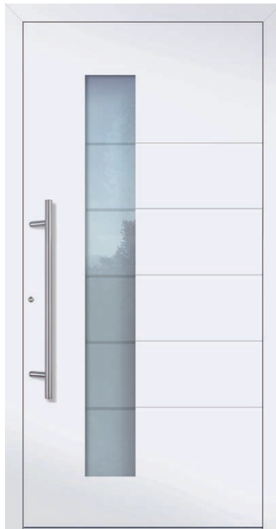
1) A 35 U_g -Wert 0,80 1) Farbe: RAL 9016 Verkehrsweiß FS Verglasung: Mattiert mit klaren Streifen LA 200 x 1.600 mm Nuten außen, 15 mm Mindestmaß = 900 x 1.990 mm
